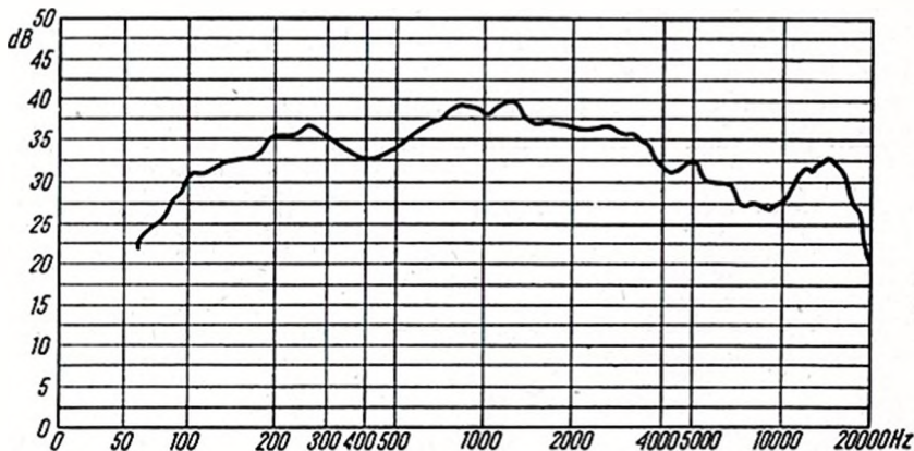
Rys. 5. Typowy przebieg charakterystyki przeniesienia zestawu głośnikowego typu GDT-8-114
