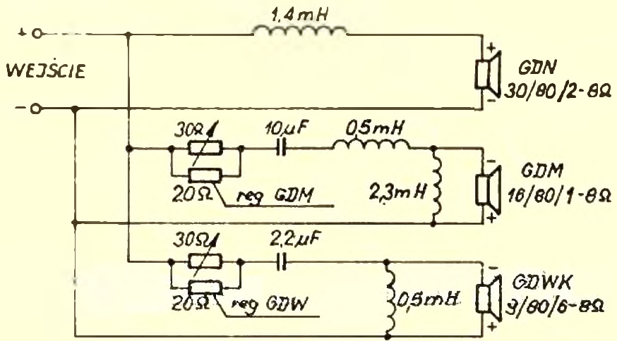
Schemat ideowy zestawu ZgB-110-8-693
