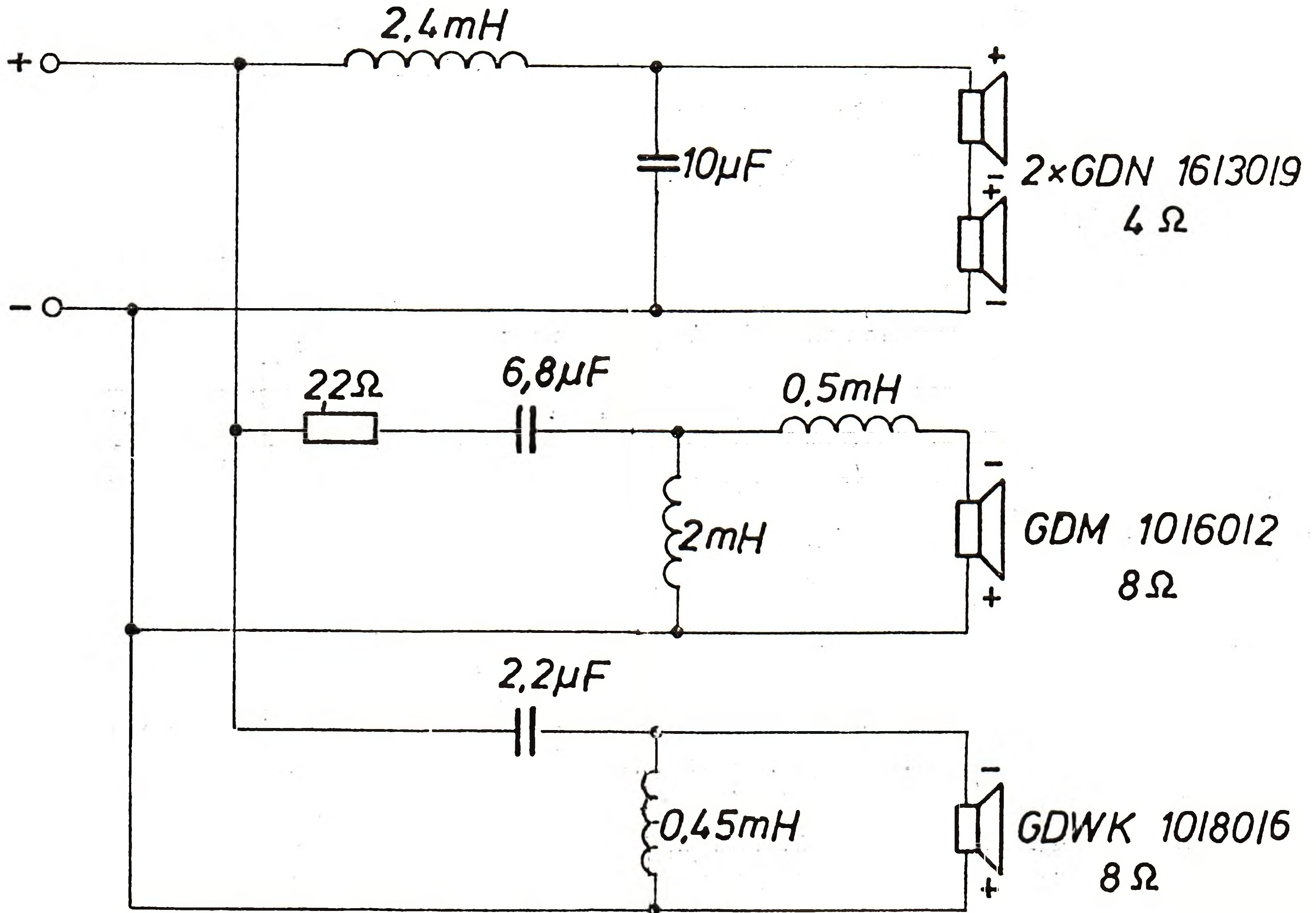
Schemat ideowy ZgR-80-8-566
