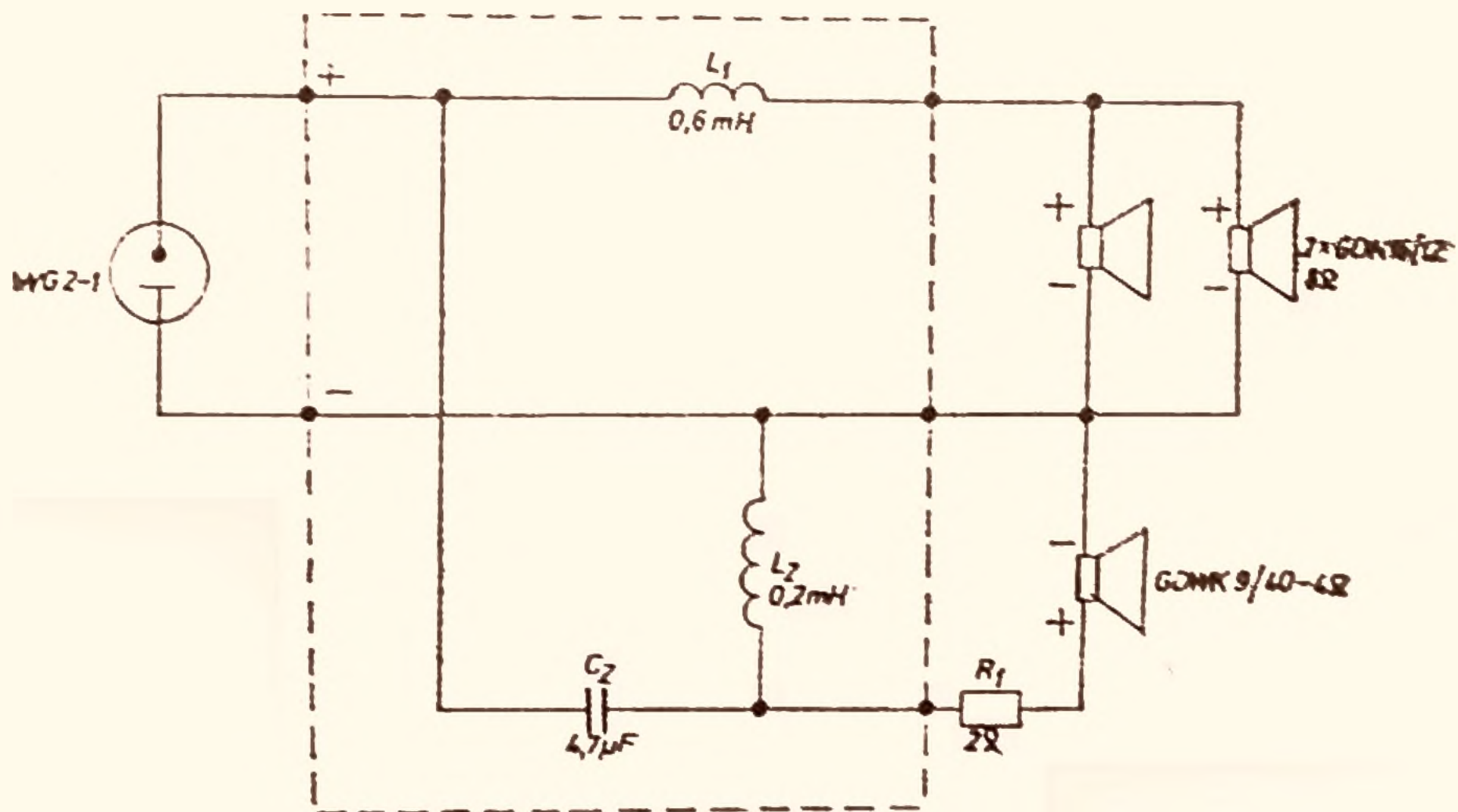
Schemat ideowy ZG25-C
