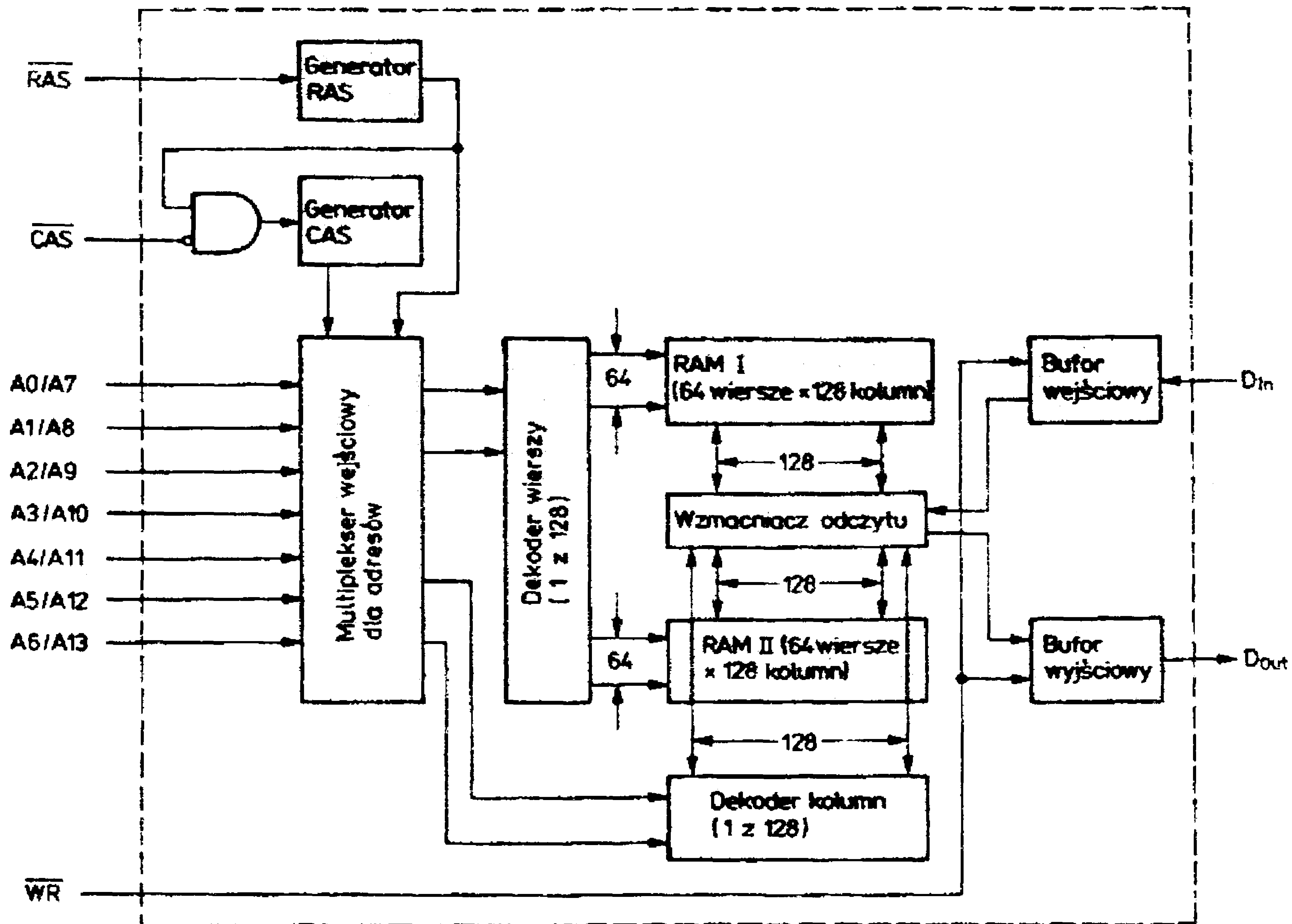
Rys. 1.37. Schemat blokowy układu pamięci 64 Kbit (typ 4164)
