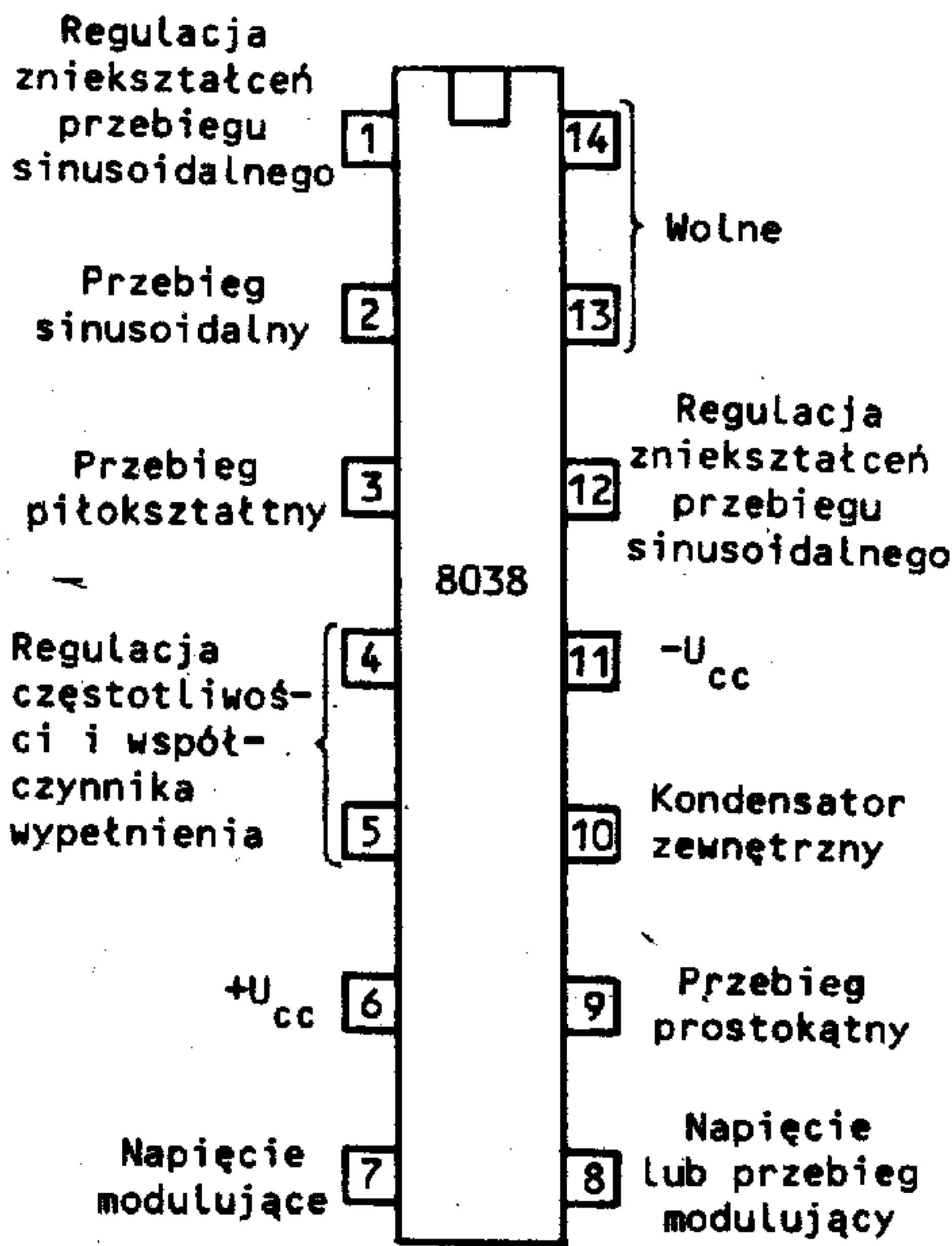
●6.22A● Uniwersalny generator funkcyjny 8038 — konfiguracja wyprowadzeń
