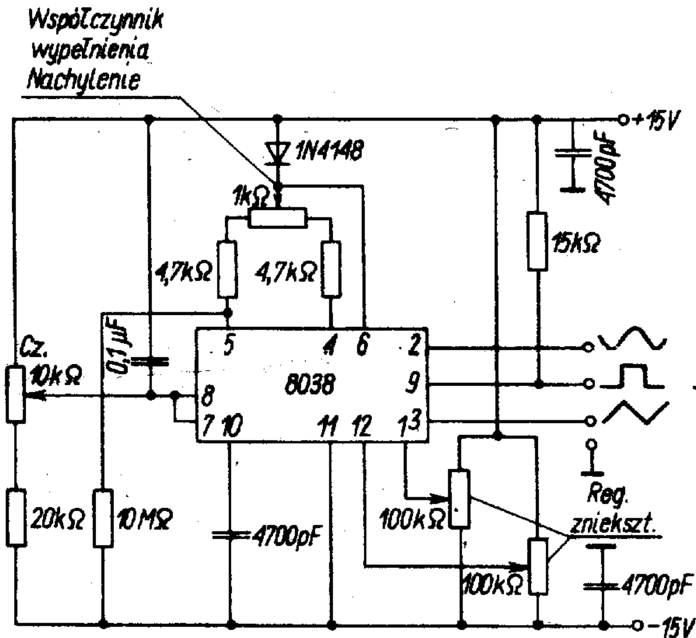
●6.22B● Układ 8038 jako uniwersalny generator akustyczny
