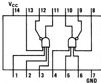
DM74H60
