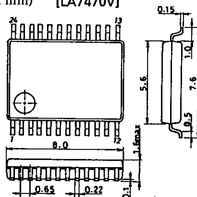
SANYO : SSOP24
