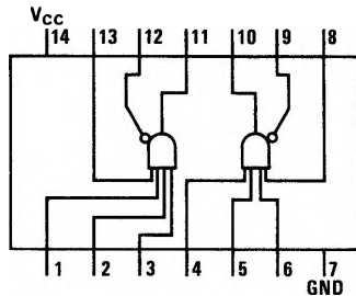
DM74H60
