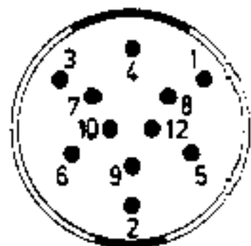
NUVISTOR
