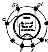
Sockelschaltenschema
