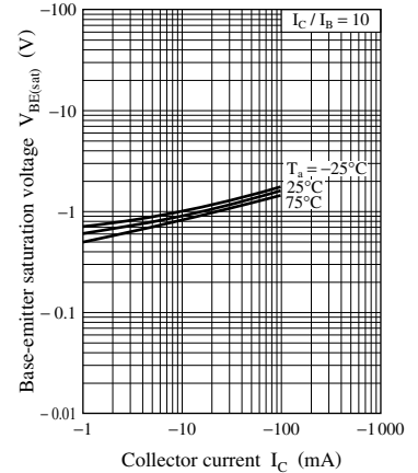
V_{BE(sat)} - I_C
