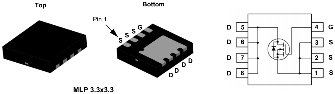
MLP 3.3x3.3
