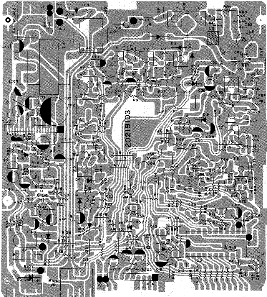
(Main P.C. Board)
