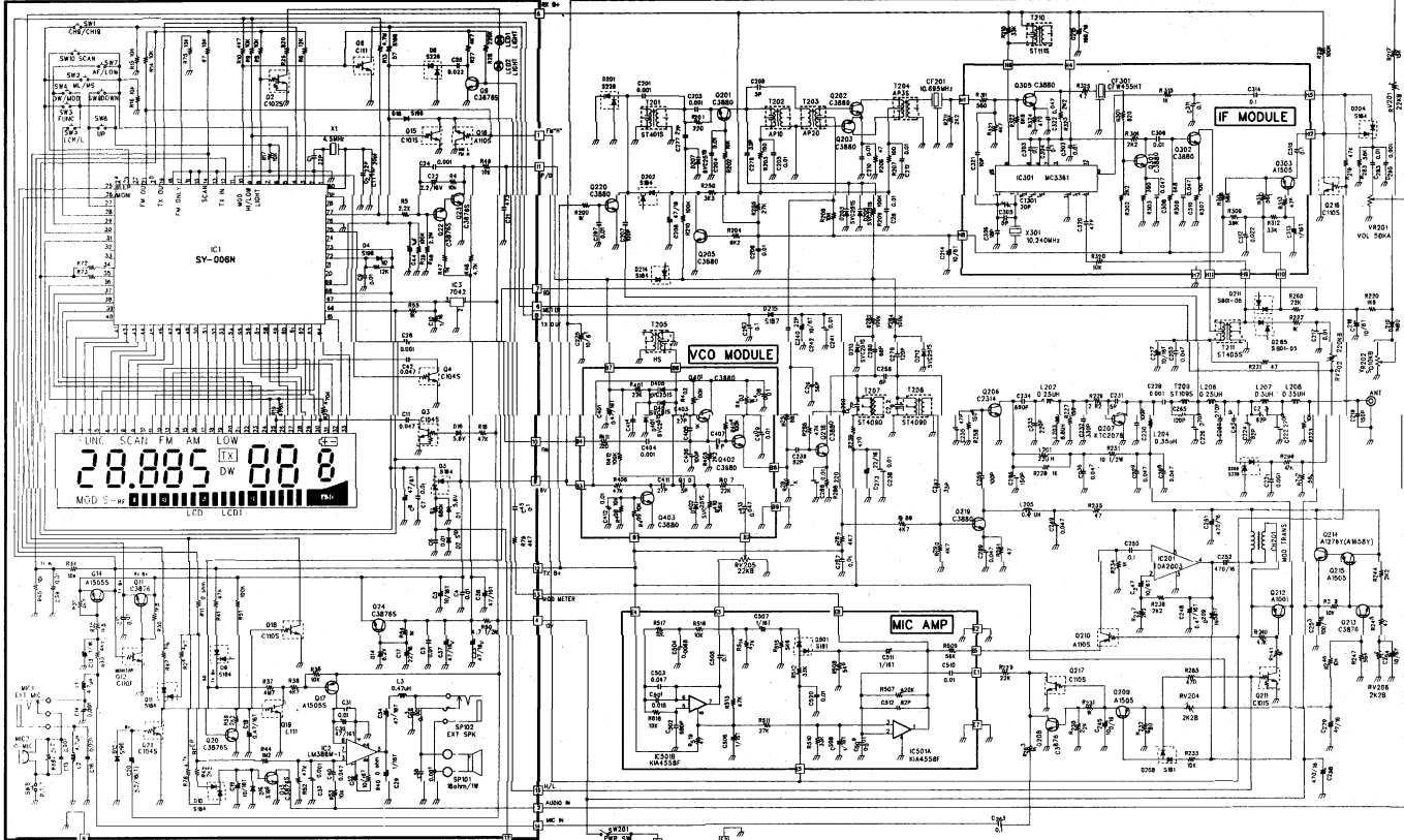
СВ радиостанция DRAGON SY-101+ UA0FKI
