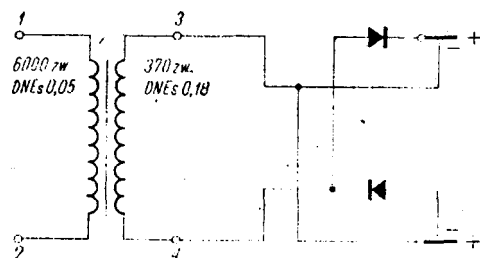
Rys. 8-66. Schemat ideowy prostownika do ładowania akumulatorów
