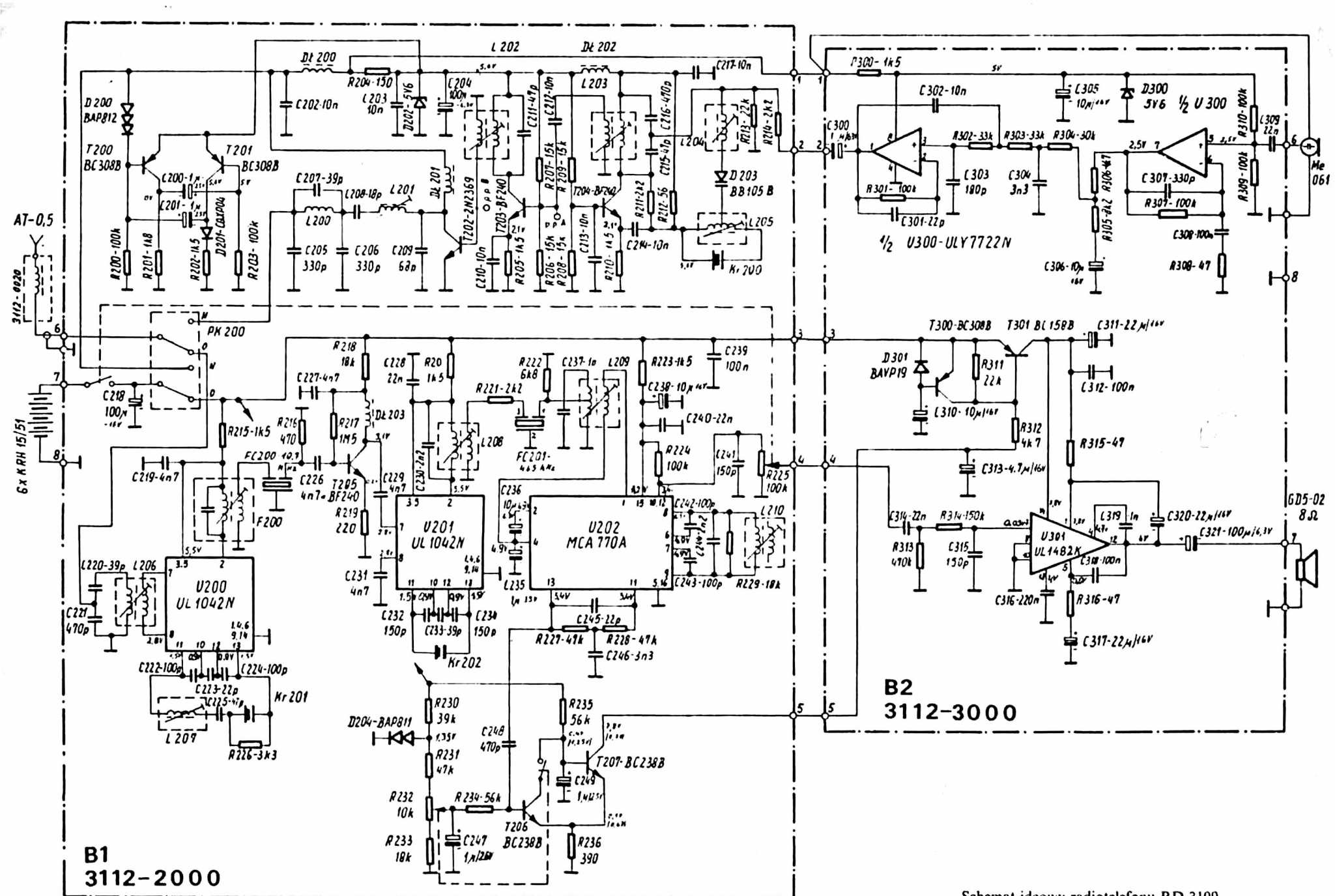
Schemat ideowy radiotelefonu RD 3109
