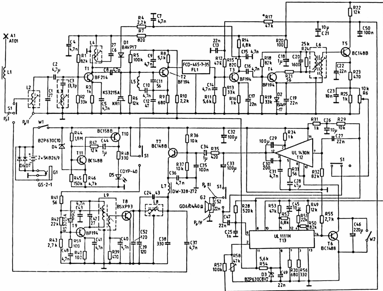
Schemat ideowy radiotelefonu Tukan
