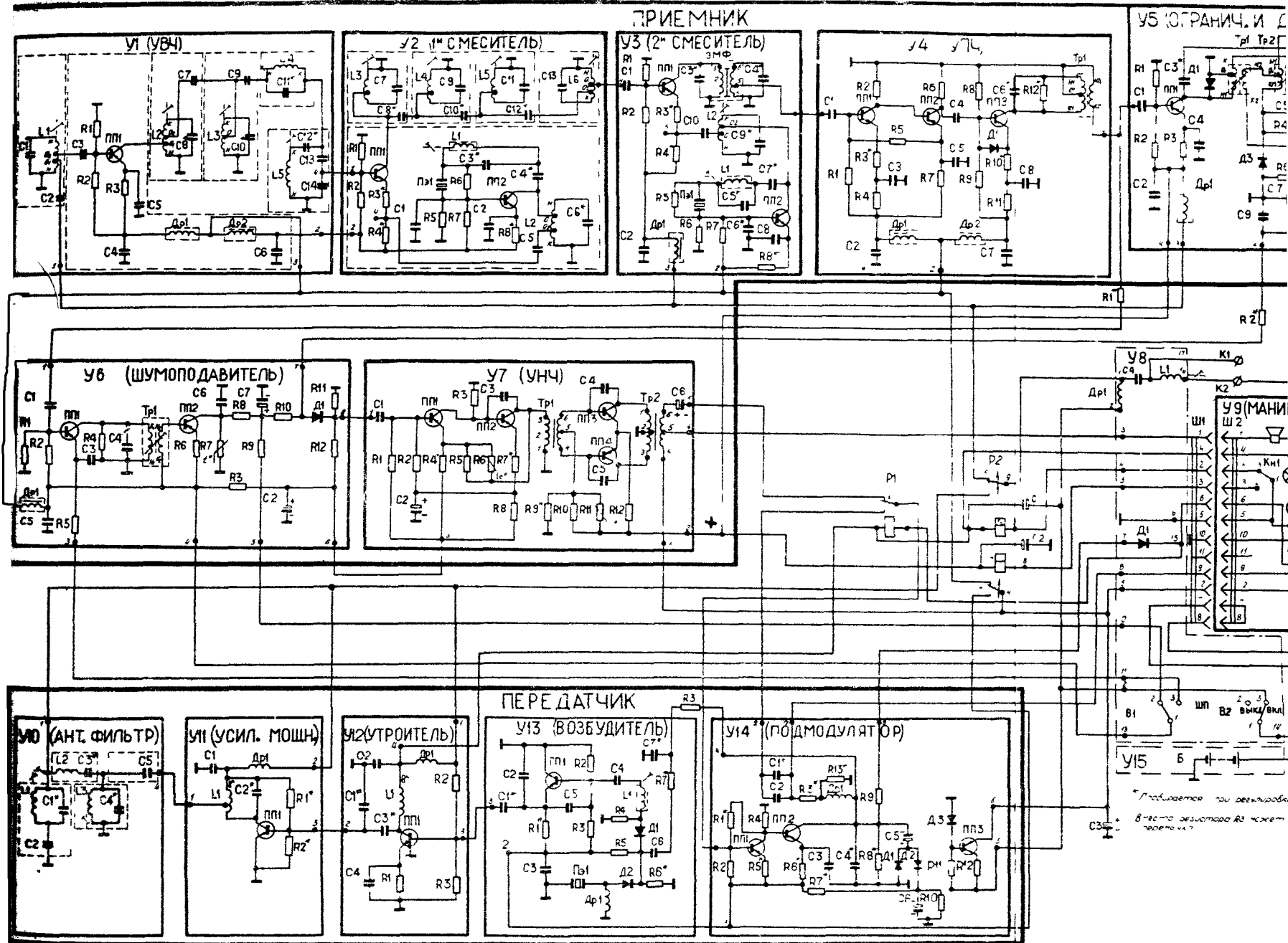
Рис 4 Схема принципиальная электрическая
