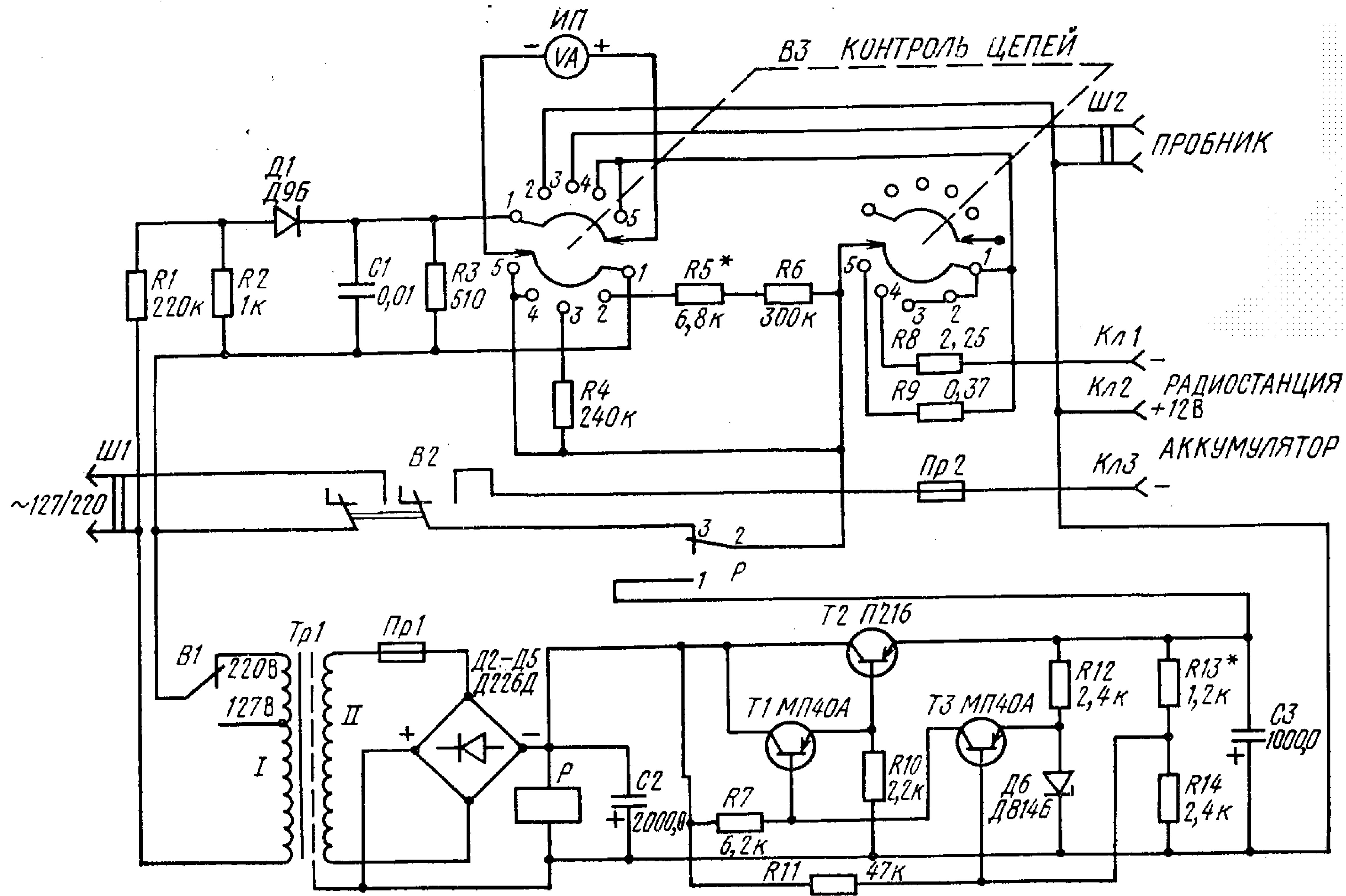
Рис. 2.8. Принципиальная схема блока питания радиостанции «Нива-М»
