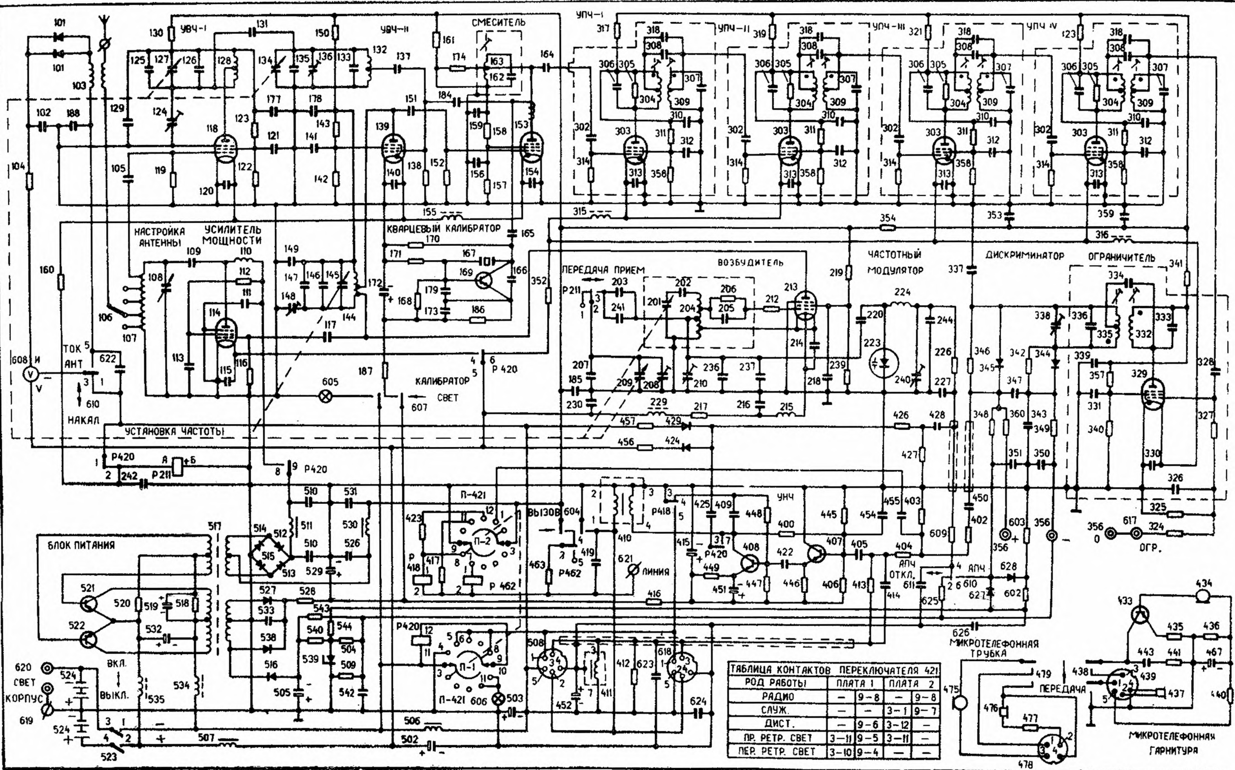
ПРИНЦИПИАЛЬНАЯ СХЕМА РАДИОСТАНЦИИ
