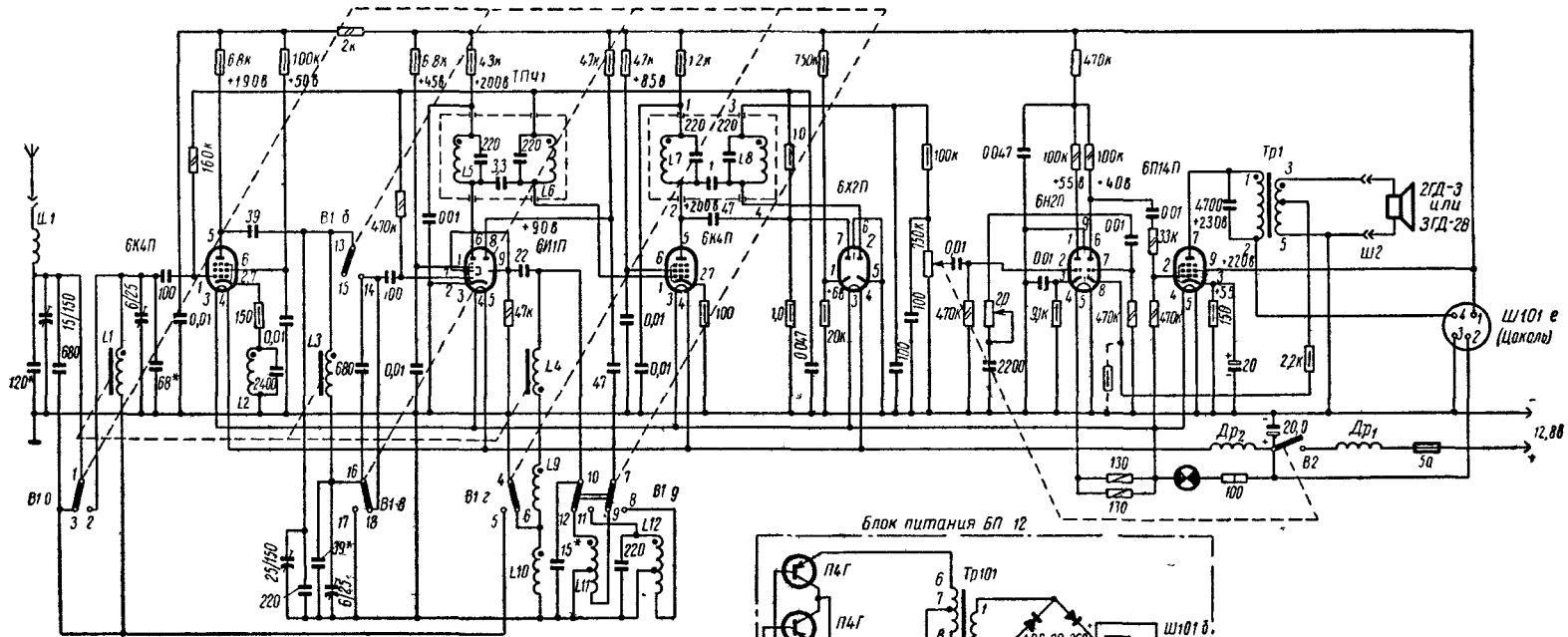
Переключатель диапазонов „В1“ показан в положении „Средние волны“
