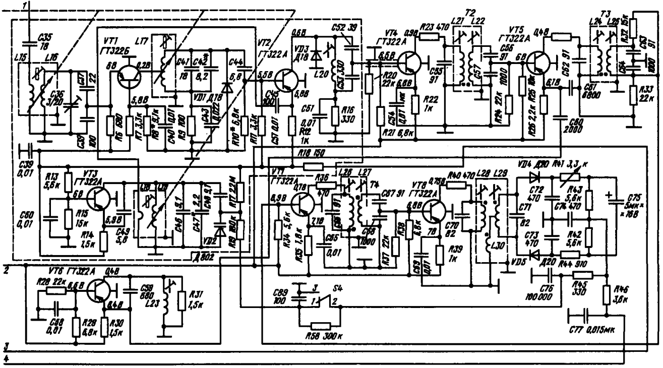
Принципиальная электрическая схема радиоприемника А-271 (А-271Г)
