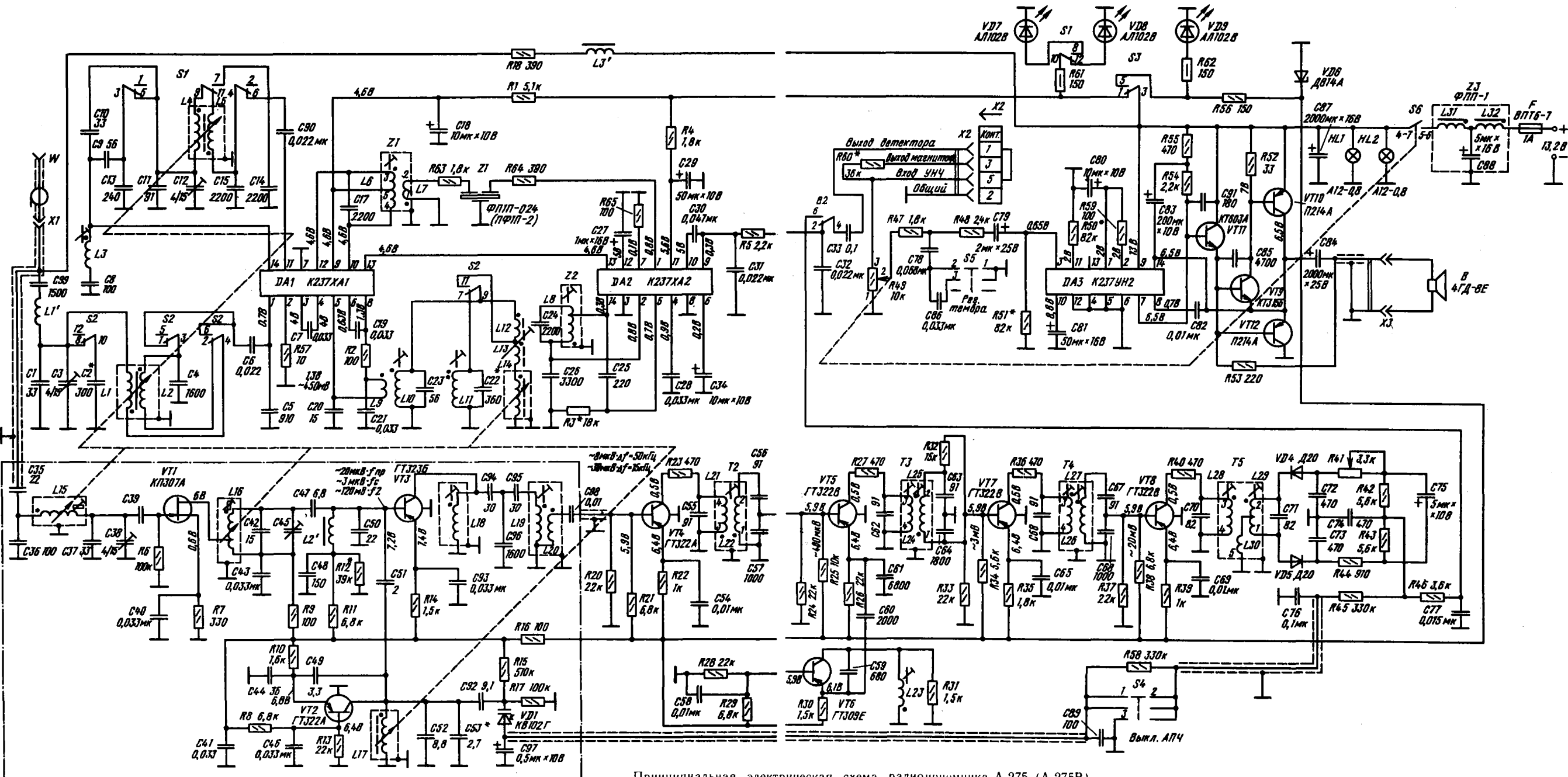
Принципиальная электрическая схема радиоприемника А-275 (А-275В)
