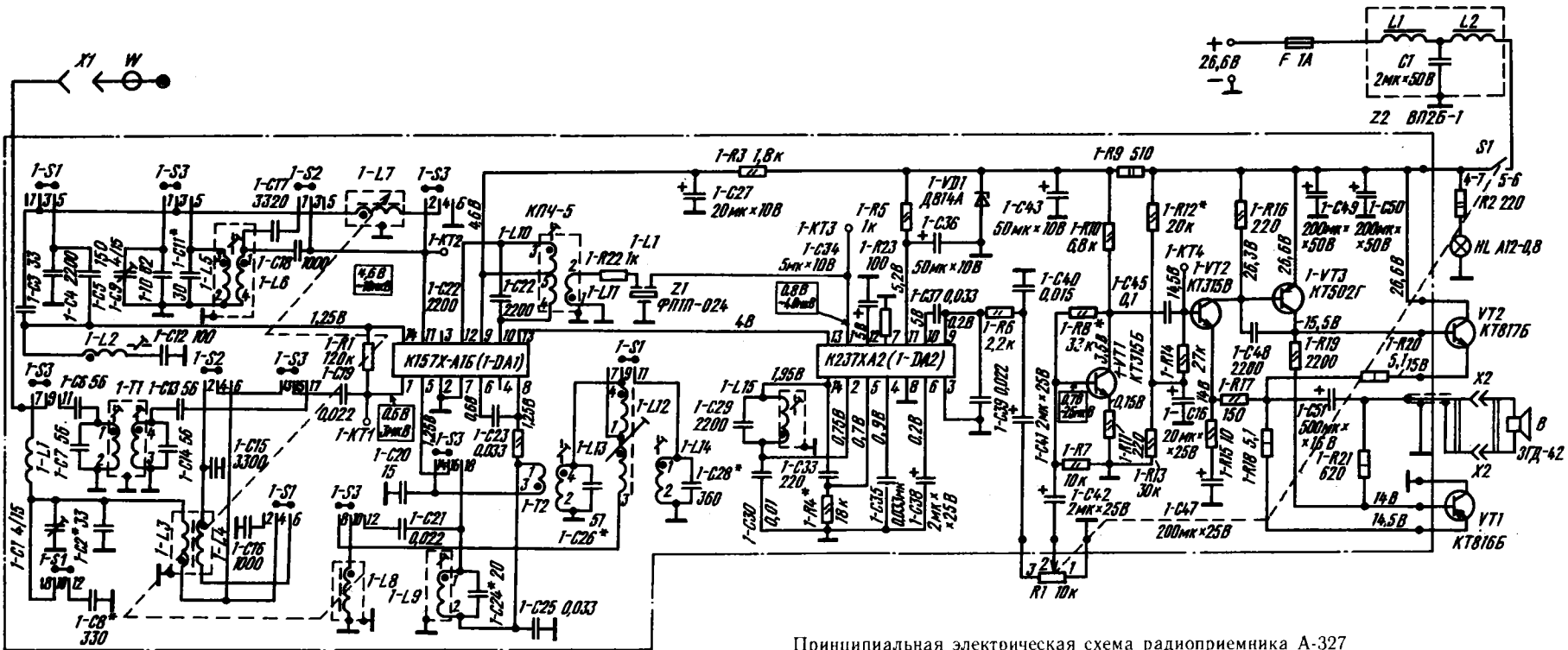
Принципиальная электрическая схема радиоприемника А-327
