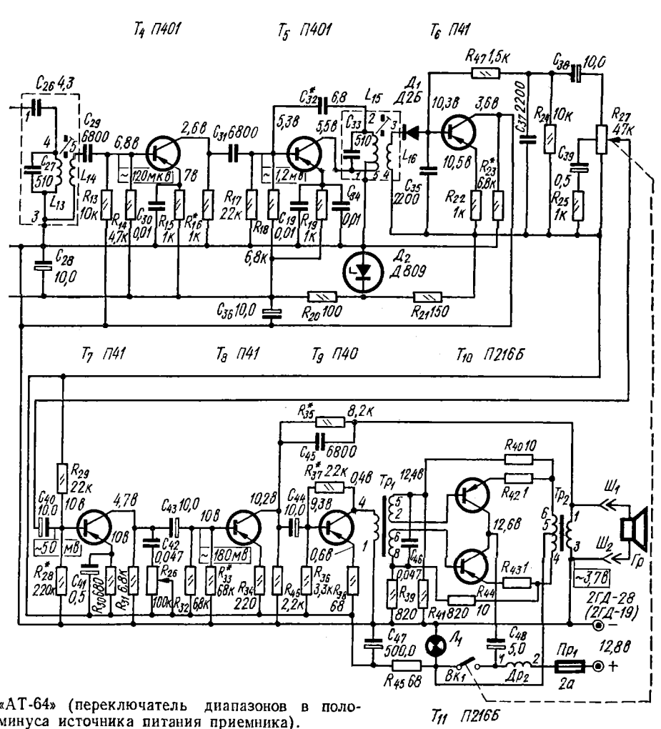
Принципиальная электрическая схема радиоприемника модели ДВ; напряжения измерены относительно
