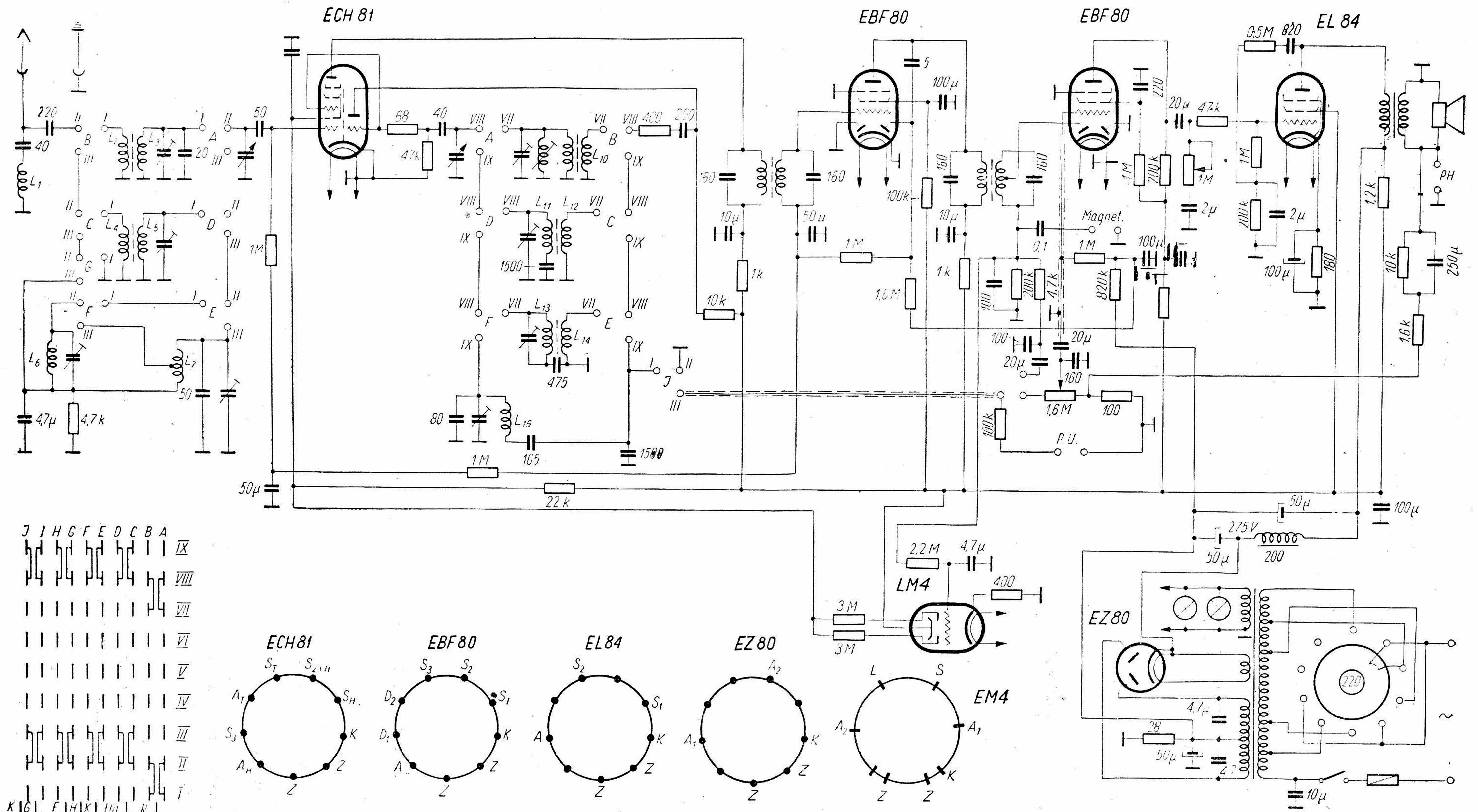
Schemat ideowy odbiornika BALATON-R656
