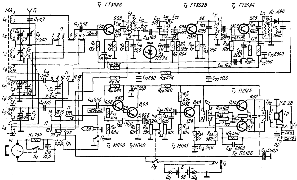
Принципиальная электрическая схема радиолы «Бригантина» (переключатель диапазонов в положении ДВ).
