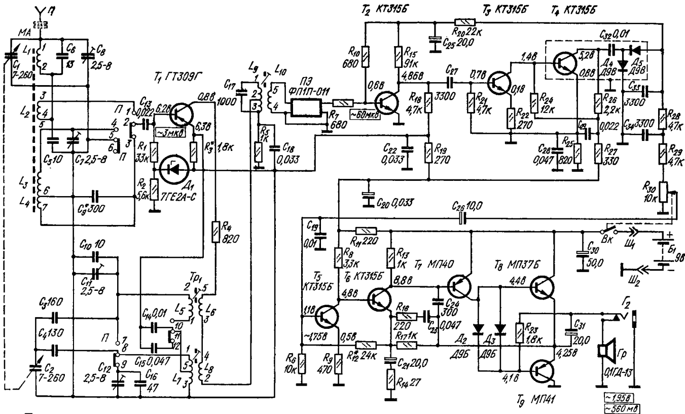
Принципиальная электрическая схема радиоприемников «Этюд-603» (переключатель диапазонов в положении ДВ).
