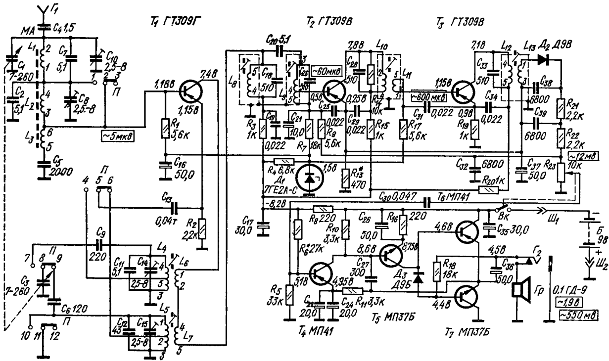
Принципиальная электрическая схема радиоприемников «Этюд» (переключатель диапазонов в положении ДВ).
