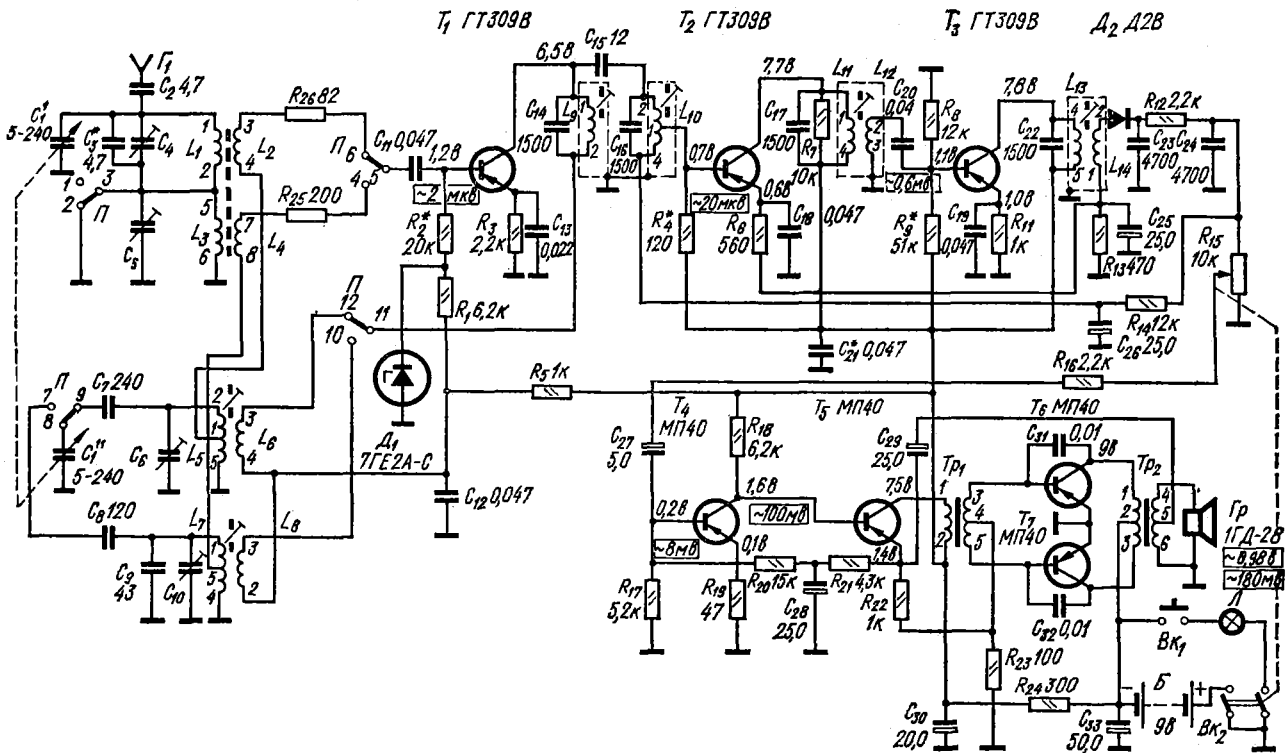
Принципиальная электрическая схема радиоприемника «Гяла» (переключатель диапазонов в положении СВ).
