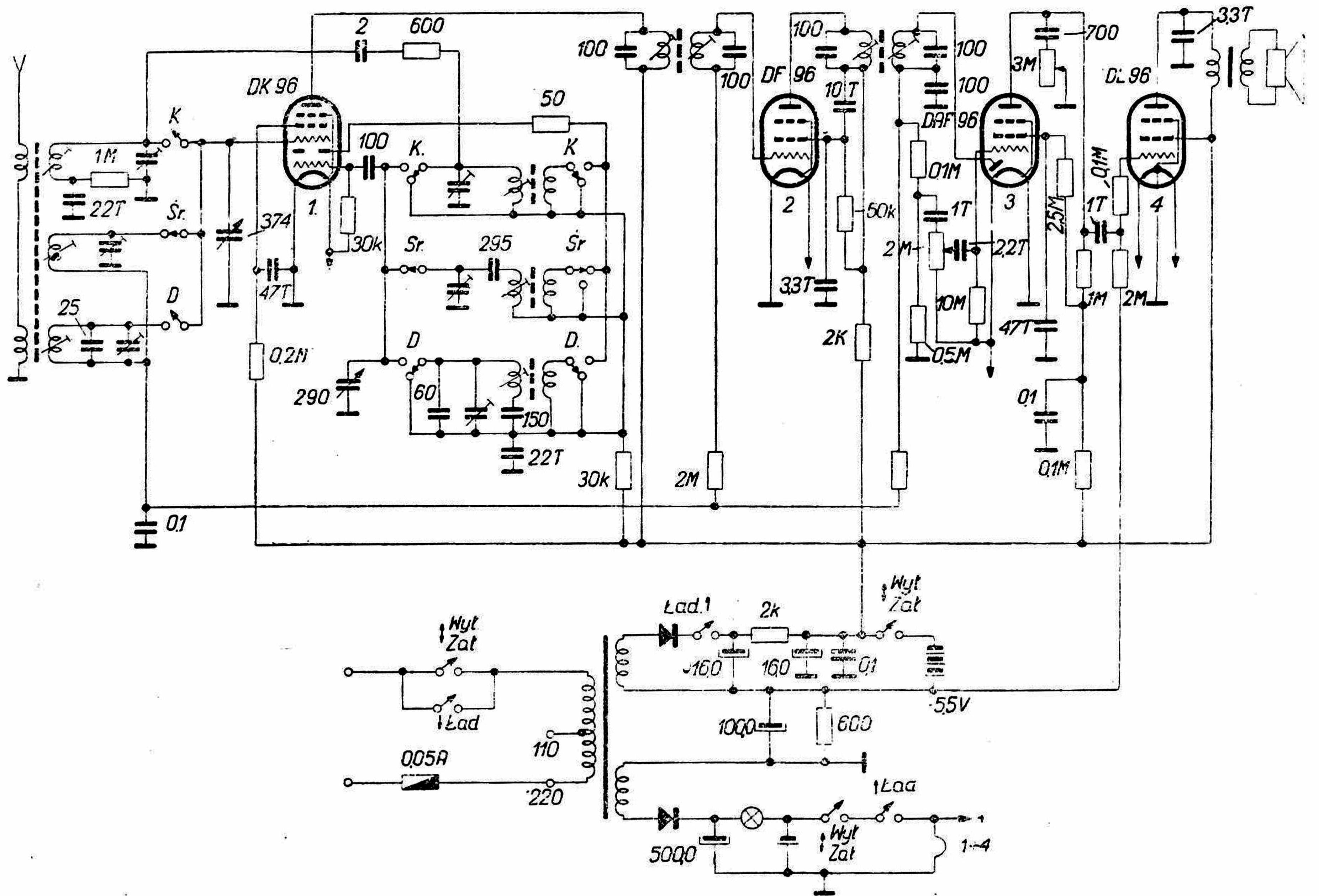
Rys. 1. Schemat ideowy odbiornika Grundig Drucktasten Boy 56
