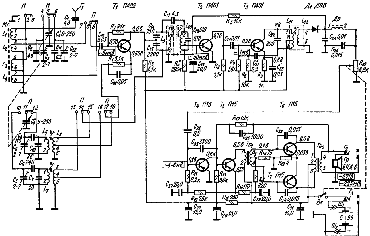
Принципиальная электрическая схема радиоприемника «Киев-7» (переключатель диапазонов в положении ДВ).
