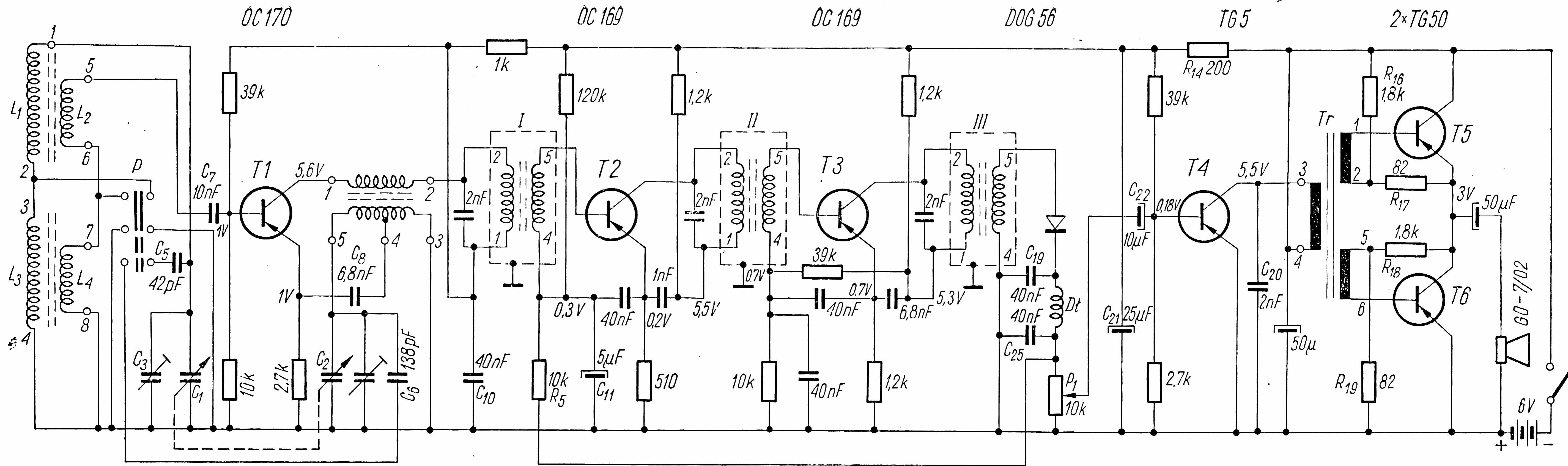
Schemat ideowy odbiornika „Koliber 2”
