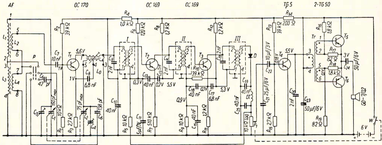
Schemat ideowy odbiornika „Koliber 2”
