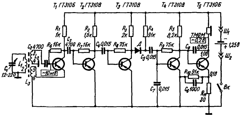
Принципиальная электрическая схема радиоприемников «Маяк-1а» и «Эра-2М».
