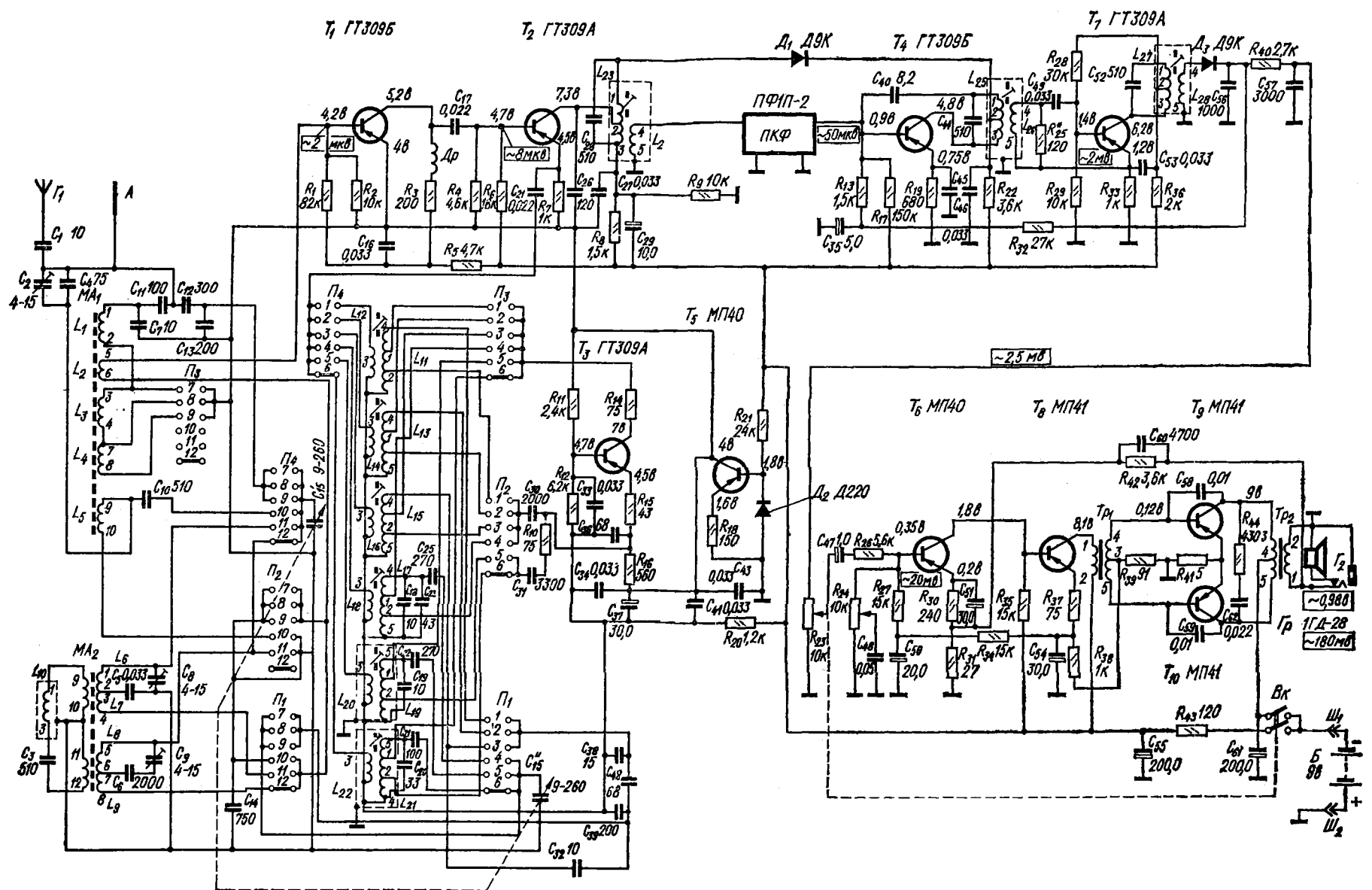
Принципиальная электрическая схема радиоприемника «Меридиан» (переключатель диапазонов в положении ДВ).
