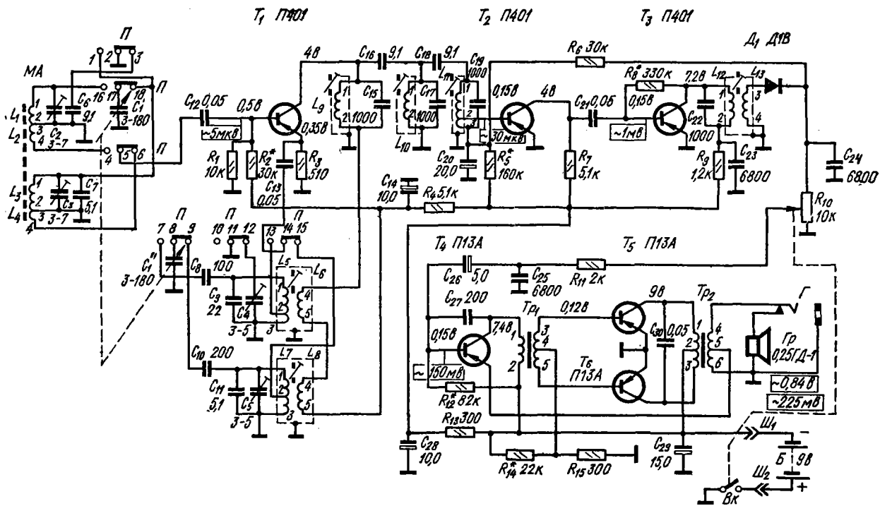
Принципиальная электрическая схема радиоприемника «Мир» (переключатель диапазонов в положении СВ).
