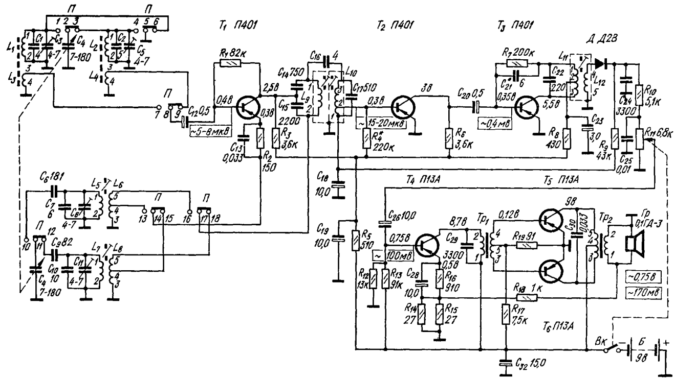
Принципиальная электрическая схема радиоприемников «Нева» и «Чайка» (переключатель диапазонов в положении СВ).
