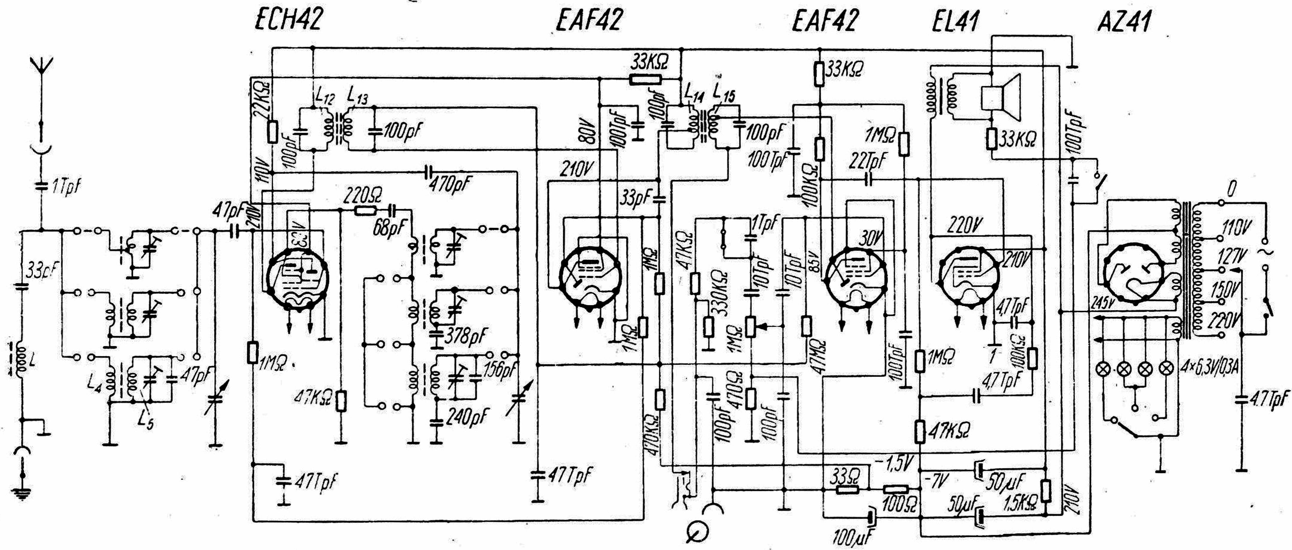
Schemat ideowy odbiornika Qualiton A 814
