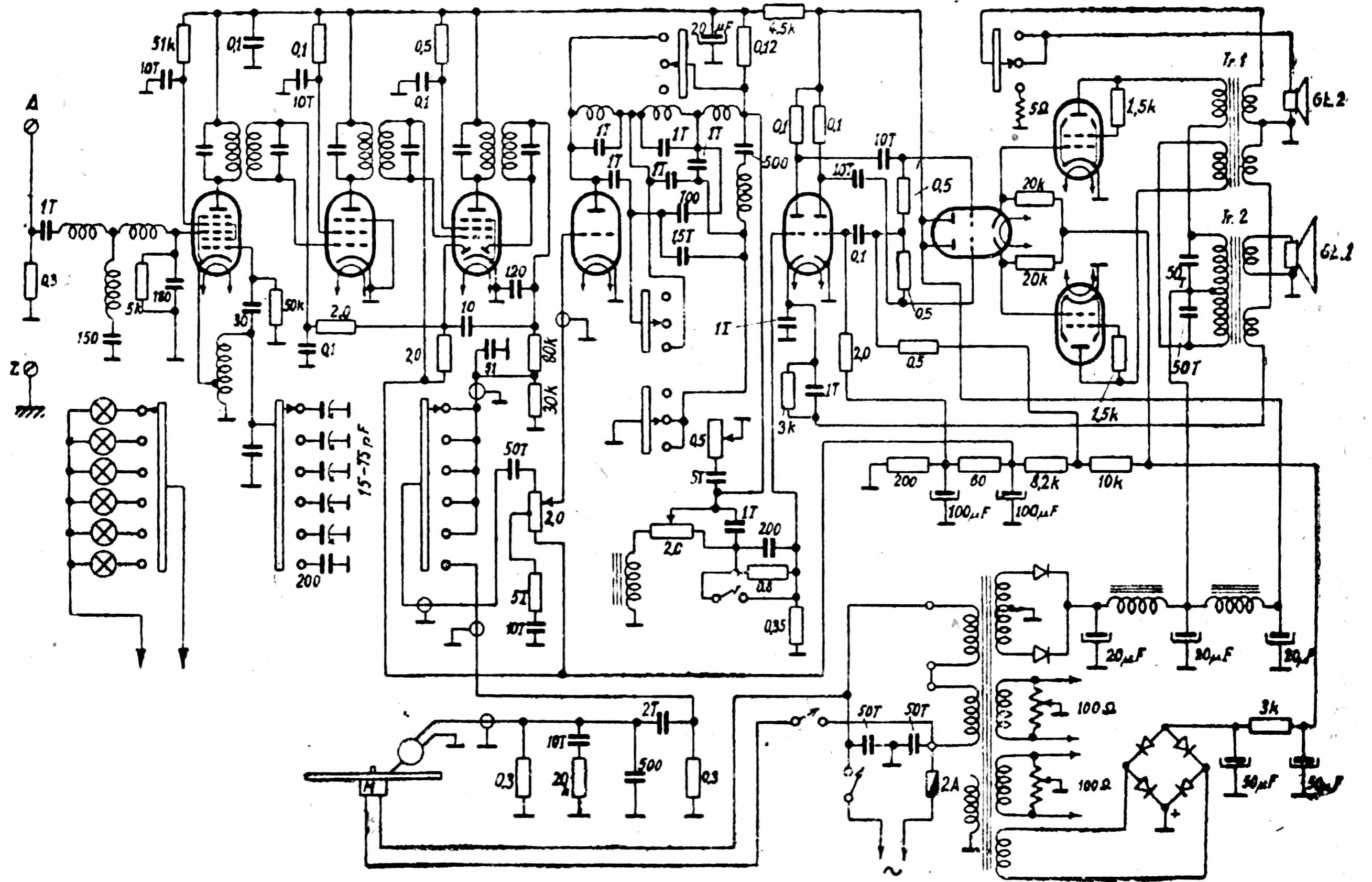
Schemat radiogramofonu W. W. Czerniawskiego
