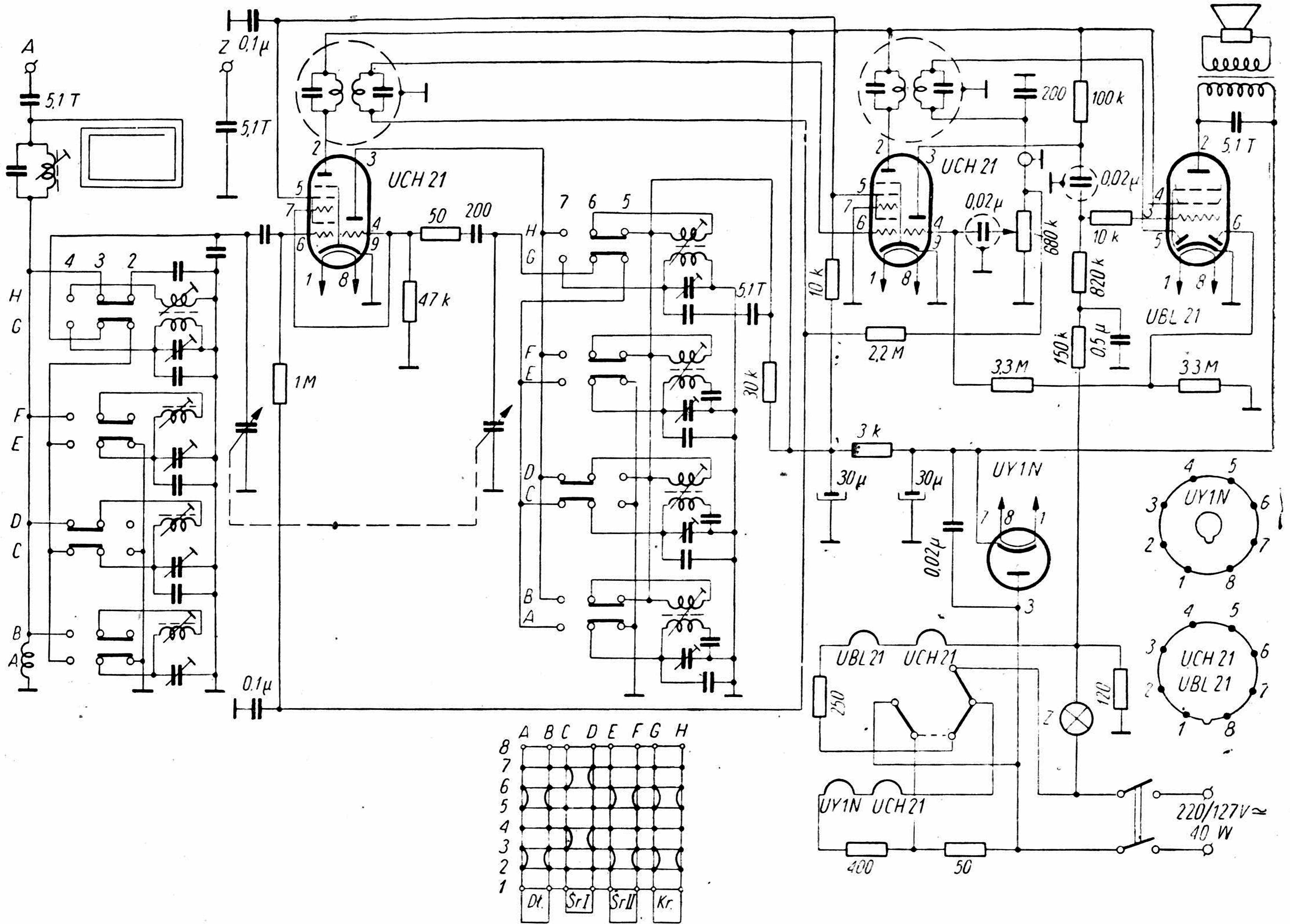
Schemat ideowy odbiornika „Sonatina“
