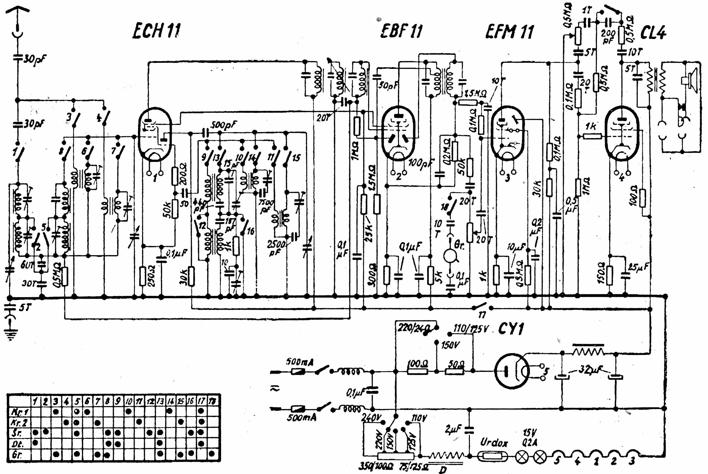
Schemat odbiornika Saba 458 GWK.
