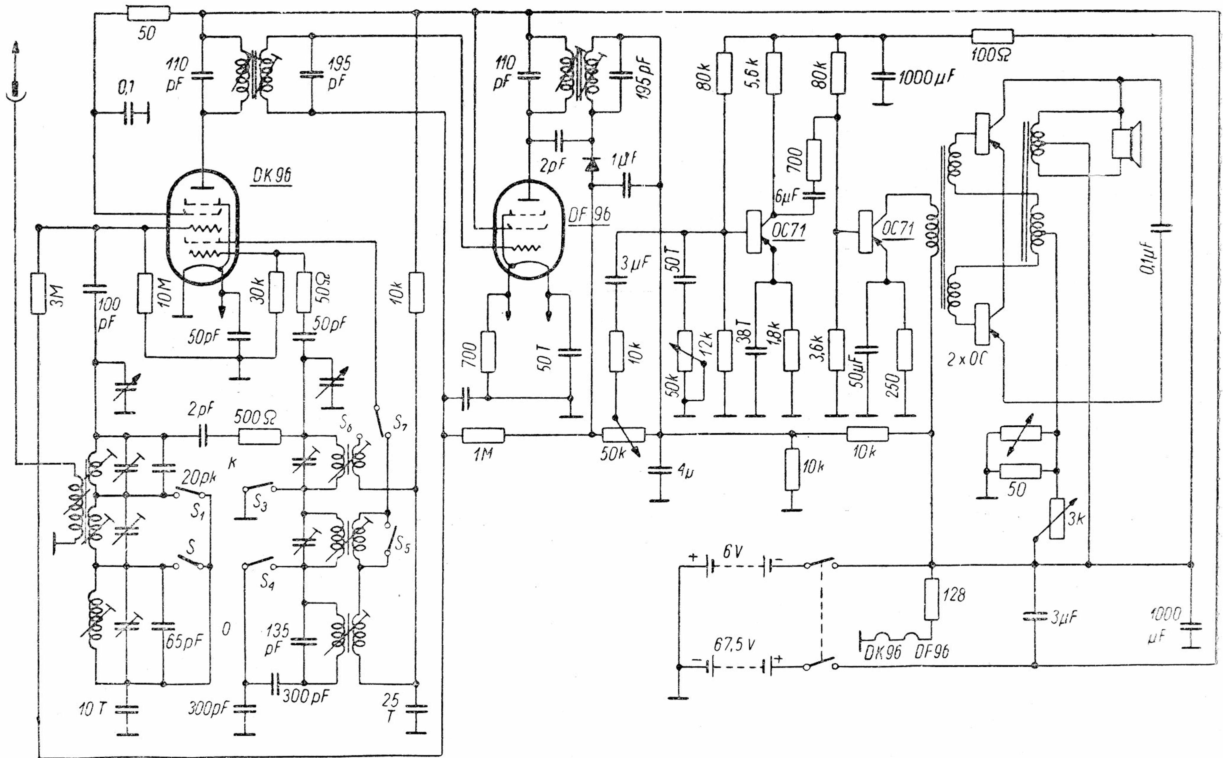
Schemat ideowy odbiornika „Bambi“ firmy Schaub Lorenz
