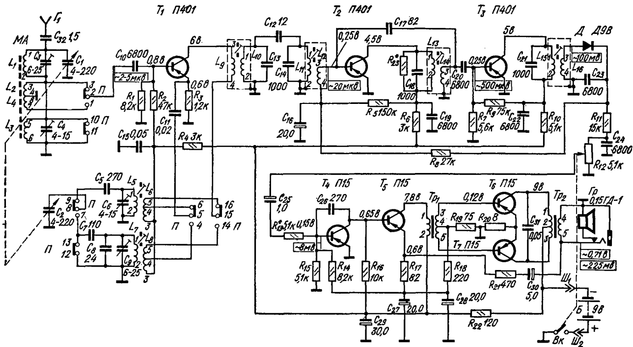
Принципиальная электрическая схема радиоприемника «Селга» (переключатель диапазонов в положении СВ).
