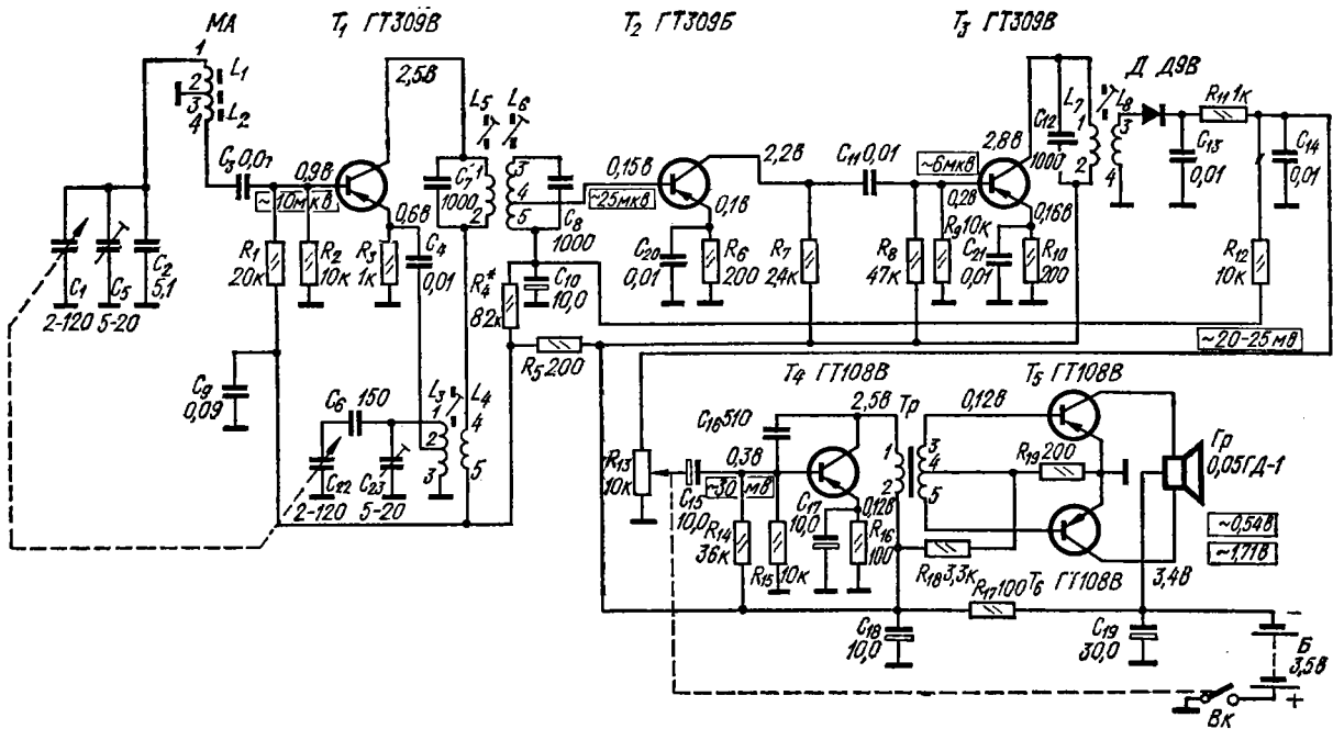
Принципиальная электрическая схема радиоприемника «Сюрприз» (вариант с диапазоном СВ).
