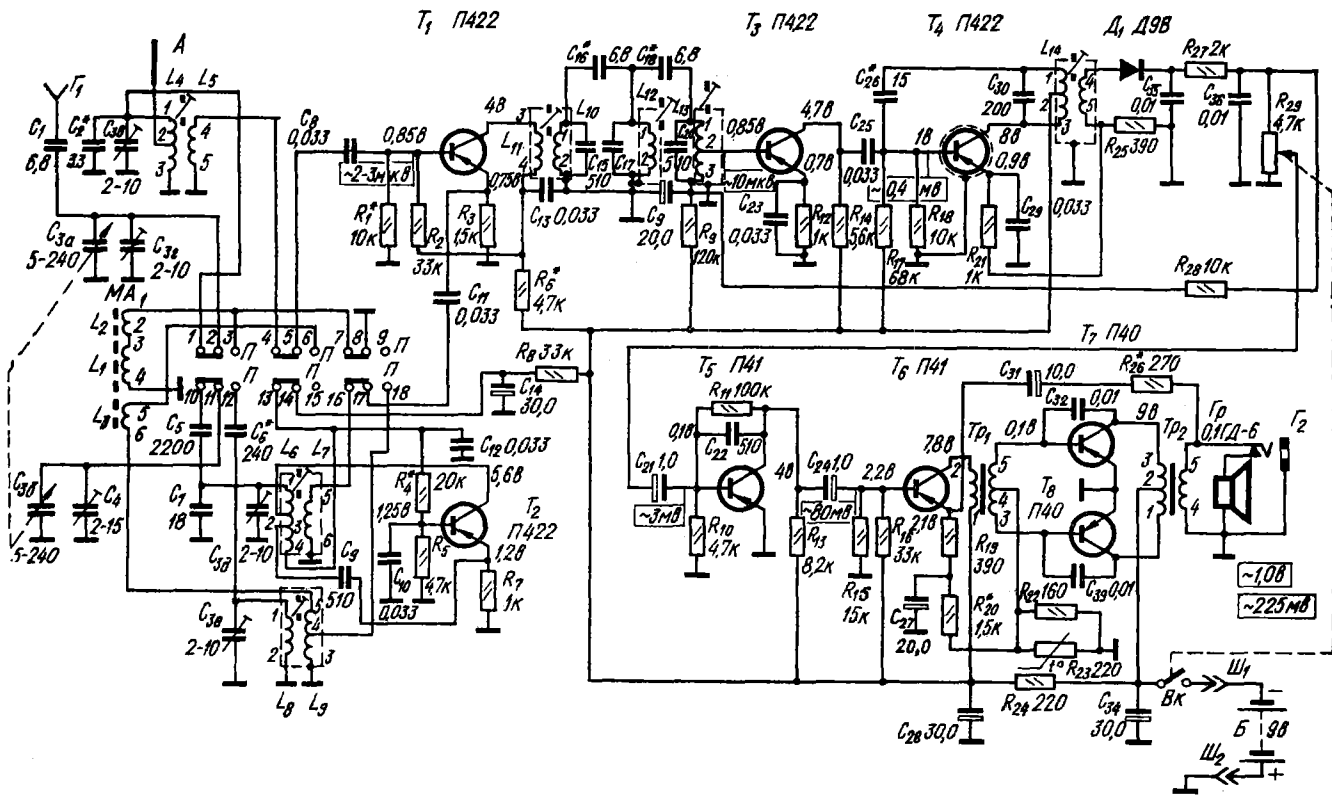
Принципиальная электрическая схема радиоприемника «Сокол-2» (переключатель диапазонов КВ).
