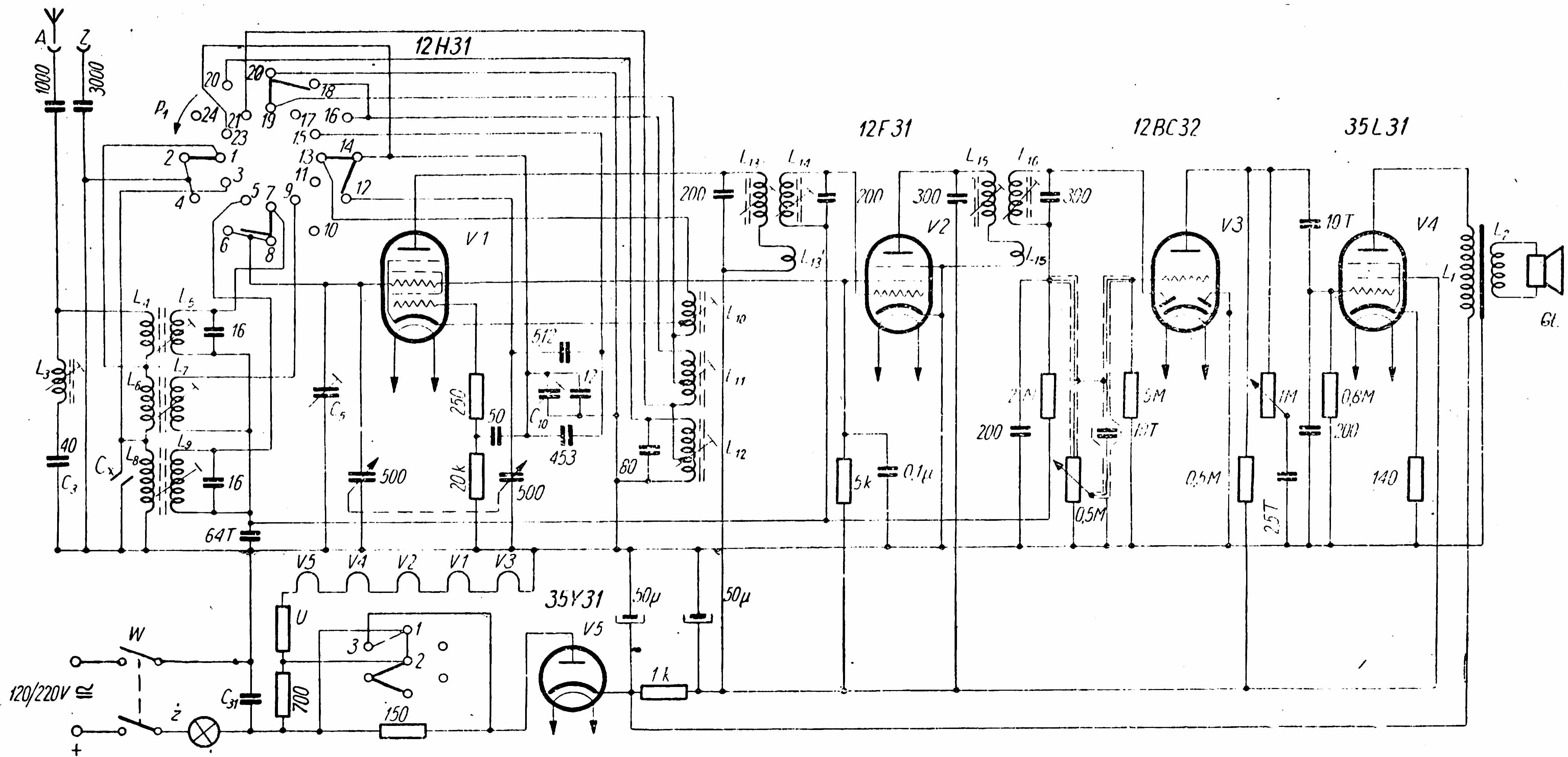
Rys. 1. Schemat ideowy odbiornika Tesla 420 U
