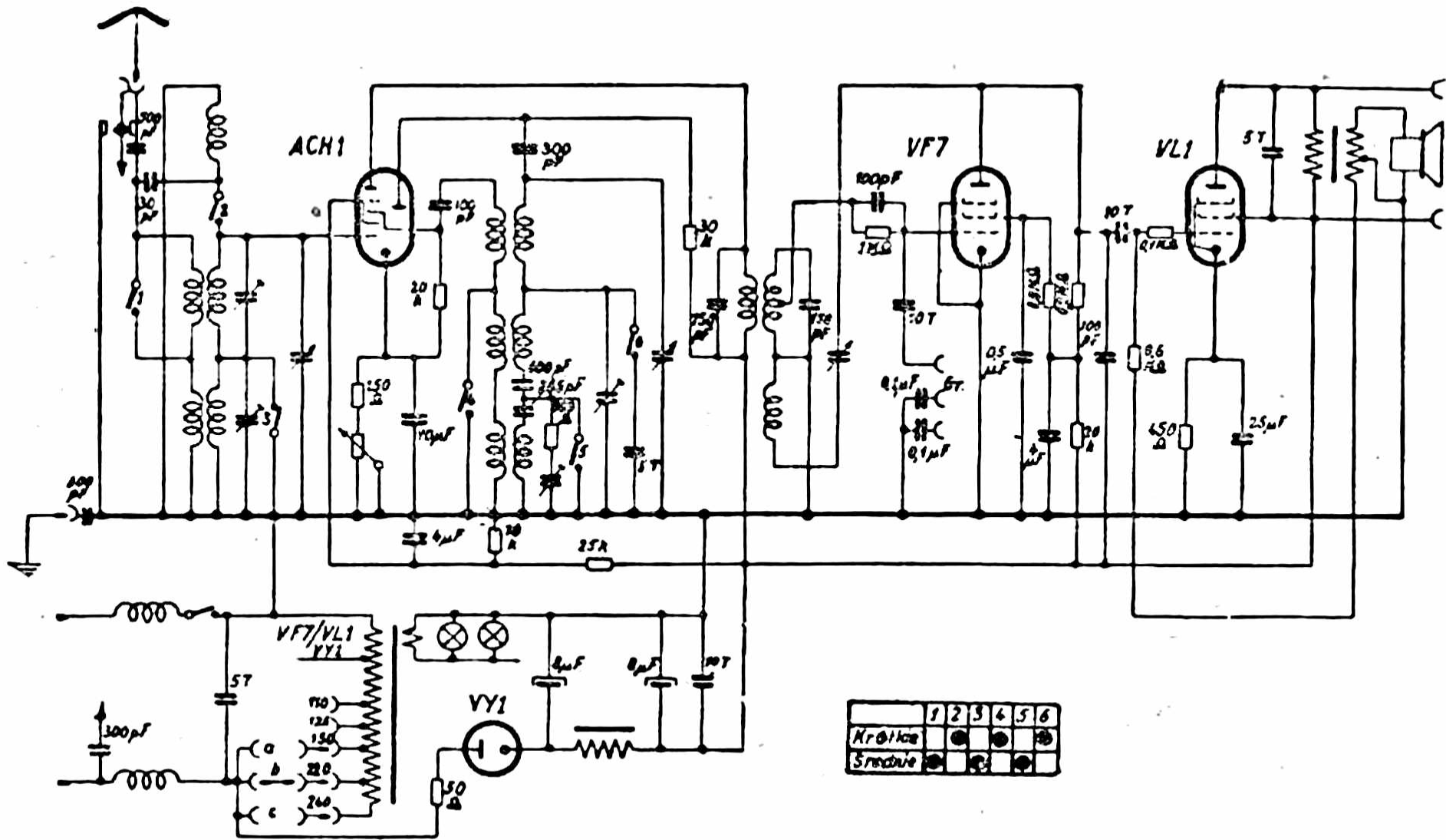
„TELEFUNKEN T4Z“
