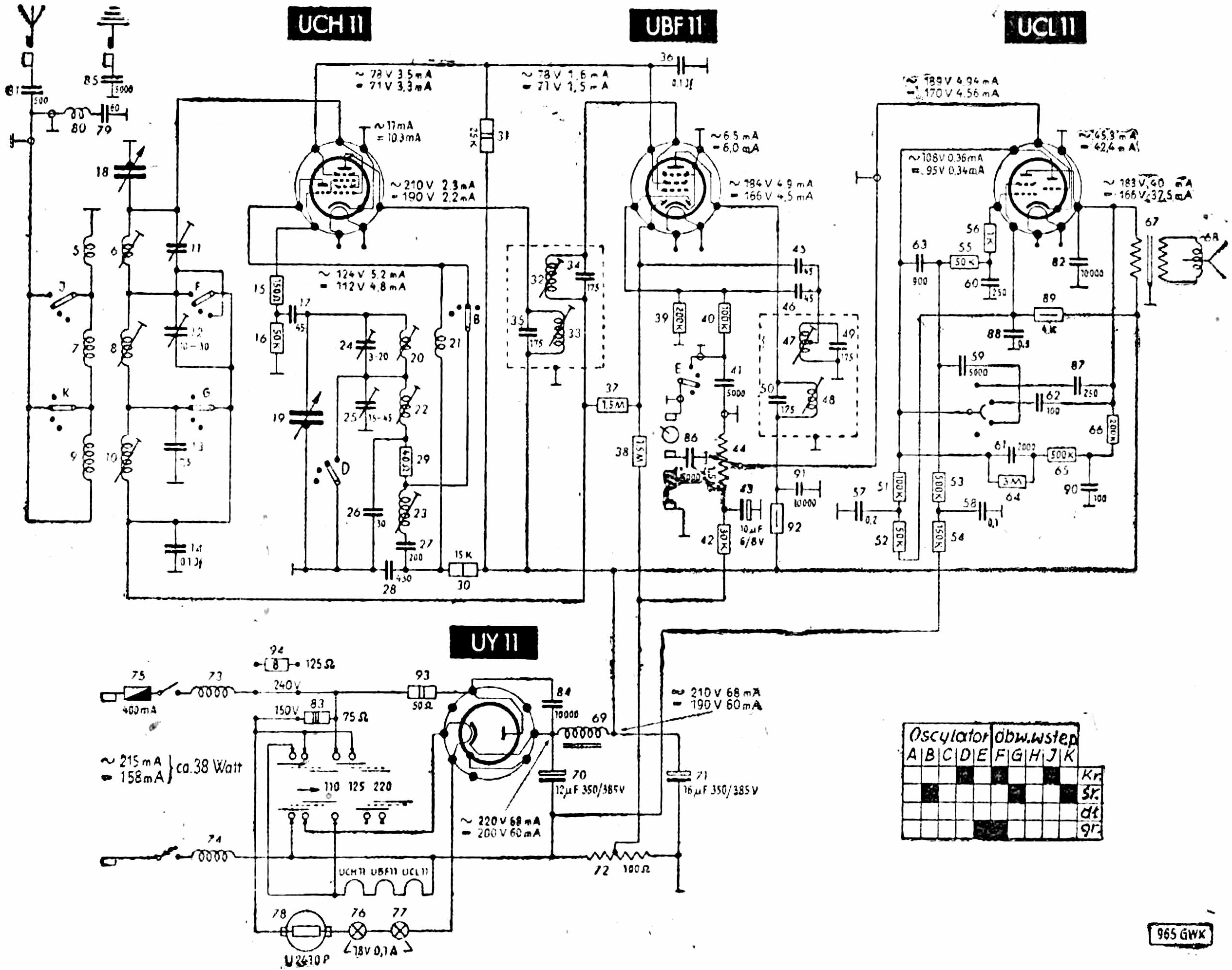
Schemat odbiornika Telefunken 965 GWK.
